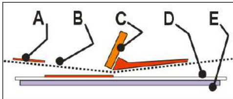
Imagen 326 Impresion con altura malla-soporte A: Tinta en la malla B: Malla C: Goma de la raqueta D: Tela a estampar E: Paleta de impresión
