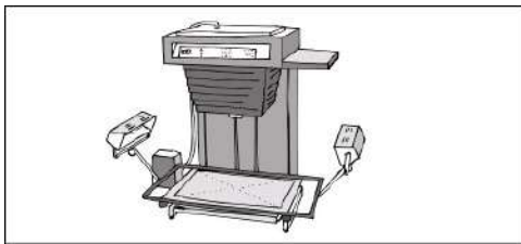
Imagen 053_02 Cámara vertical para fotomecánica
