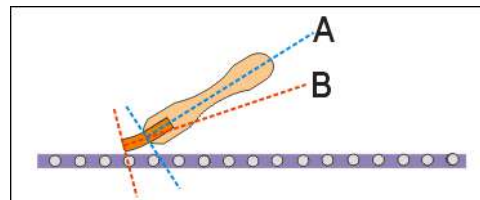
Imagen 510_01 A Angulo de la racleta B Angulo del filo de la goma
