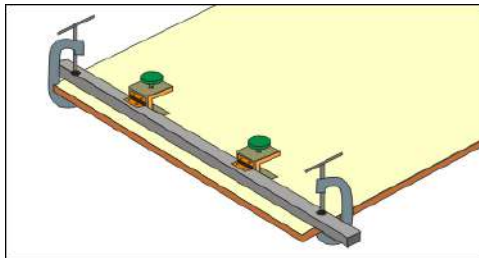
Imagen 453_04 Prensas abisagradas desplazables
