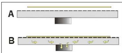
Imagen 418_01 A: Succión no activada B: Succión de vacío activada
