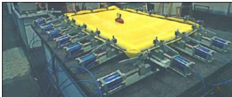
Equipo automático para el tensado de las mallas
