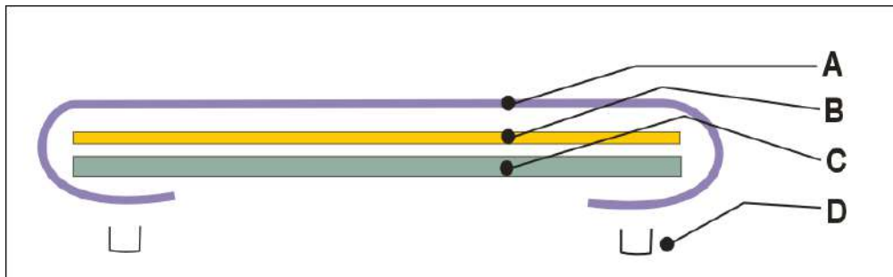
Imagen 323 Vista de perfil de un paleta de superficie blanda A: Tela vinílica tensada B: Espuma de poliuretano C: Placa de la base de la paleta D: Corchetes
