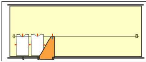
Imagen 523_10 Situando topes y marcas con la escuadra de cartón
