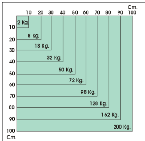
Imagen 220_02 Peso requerido por área de contacto
