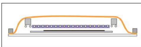
Imagen 222_02 Al bajar el marco de vacío, la lámina de goma cubre el bastidor
